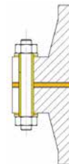
Tipo E Full Face
